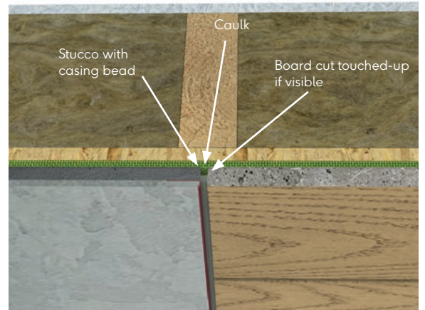
Fig.31 - Abutting stucco
